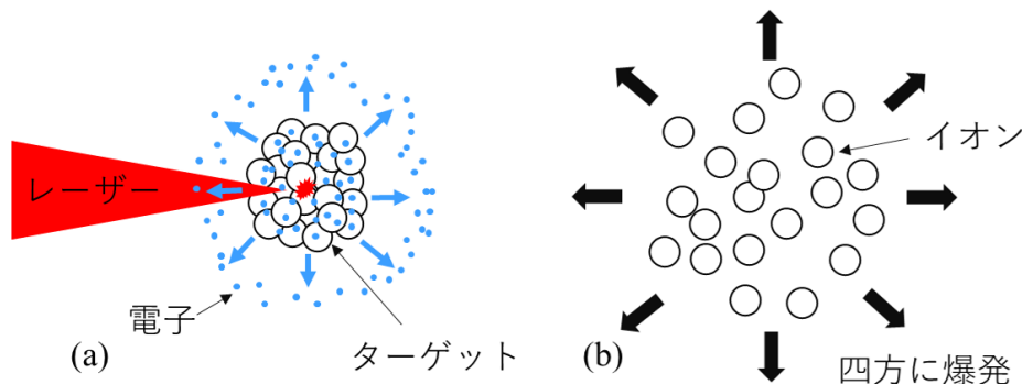
図 2 クーロン爆発によるイオン加速機構の模式図。
