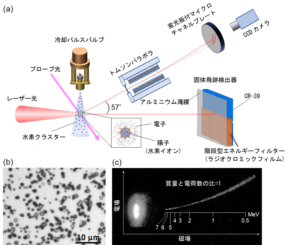
図 2. (a) 水素クラスターを用いたレーザー陽子ビーム加速実験の概略図。(b) 固体飛跡検出器（レーザー進行方向に設置）で検出されたイオンのエッチピット（腐食孔） 7) の顕微鏡画像。エッチピットの大きさから、観測されたシグナルが純度 100% の陽子ビームであることが確認されました。(c) トムソンパラボラ検出器（レーザー進行方向に対して 57 度の方向に設置）で検出された陽子ビームのエネルギー分布のシグナル。質量と電荷数の比が 1 となる唯一のイオンである陽子のみが検出されていることから、観測されたシグナルが純度 100% の陽子ビームであることが確認されました。
