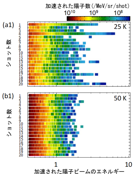
図4. (a1)温度25ケルビン、(b1)温度50ケルビンの条件で、トムソンパラボラ検出器（レーザー進行方向に対して57度の方向に設置）を用いた計測から得られた陽子ビームのエネルギースペクトル。連続する20ショットのデータを示しています。レーザー進行方向に対して57度の方向では、陽子の最大エネルギーは、温度25ケルビンの時に観測され、7.4メガ電子ボルトであることが分かりました。(a2)温度25ケルビン、(b2)温度50ケルビンの条件で、高強度レーザーと水素クラスターとの相互作用の様子を観測したシャドウグラフ画像。図中の破線で囲んだ領域がレーザーとクラスターとが強く相互作用する領域を示しています。温度25ケルビンの時には、マイクロメートルスケールの大きなサイズのクラスターとレーザーとが相互作用し、大きく丸く光る領域が存在していることがわかります。
