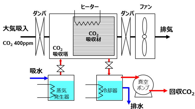
図1 DAC小型試験装置の模式図とその専用実験棟(RITE敷地内)の外観
